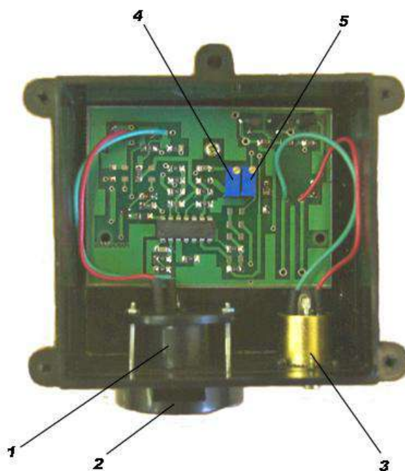
Рис.3. Датчик СИГМА-03.ДЭ со снятой крышкой.
